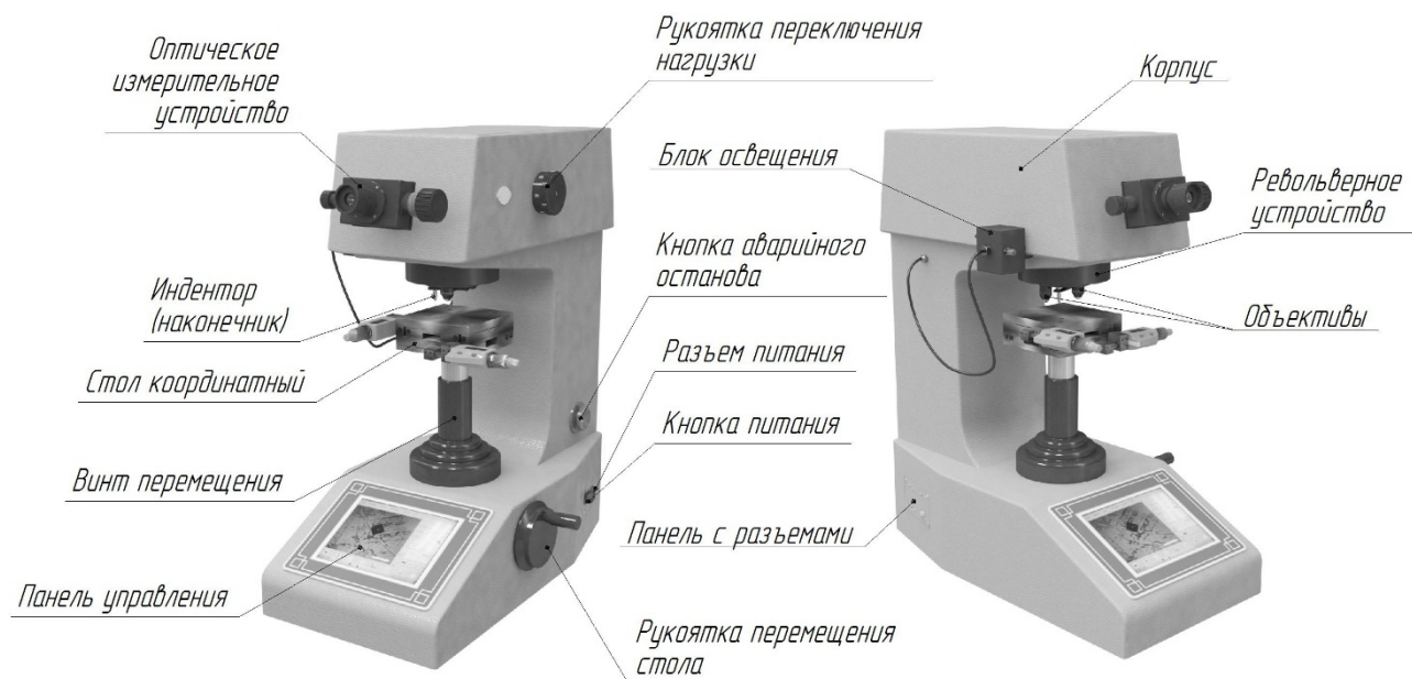
Рисунок 1 – Общий вид твердомера ИТВ-10-МЖ
